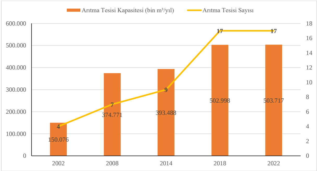
Grafik 43: İçme ve Kullanma Suyu Arıtma Tesisi Kapasitesi (bin m 3 /yıl) ve Sayısı
