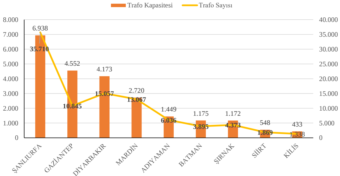
Grafik 48: İllere Göre Dağıtım Gerilim Seviyesindeki Trafo Kapasiteleri ve Trafo Sayıları (2024)
